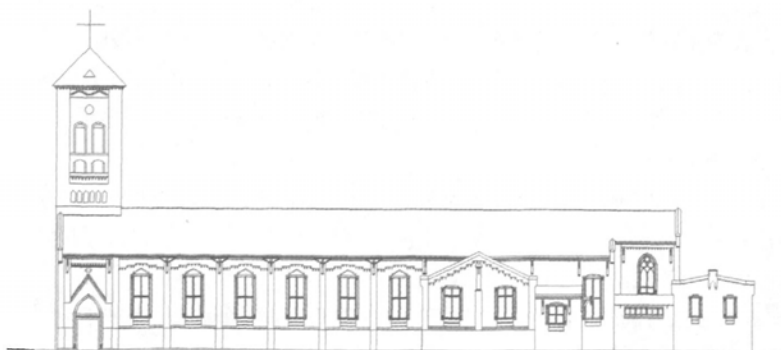
图5 主教堂东立面测绘图
