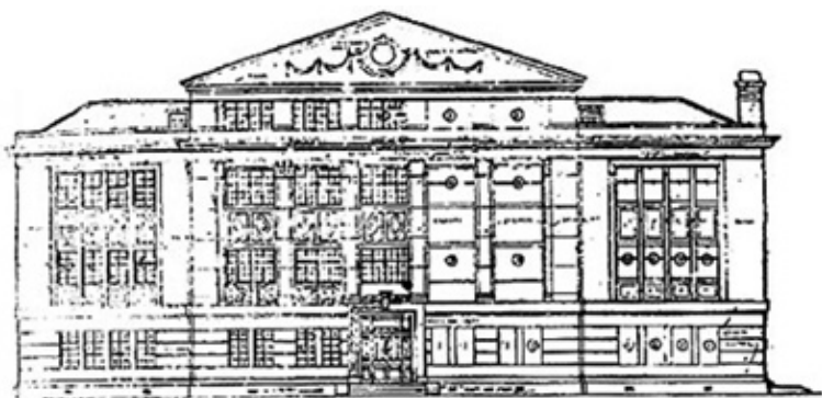
图 4.18 庚午楼正立面图（原设计图）
