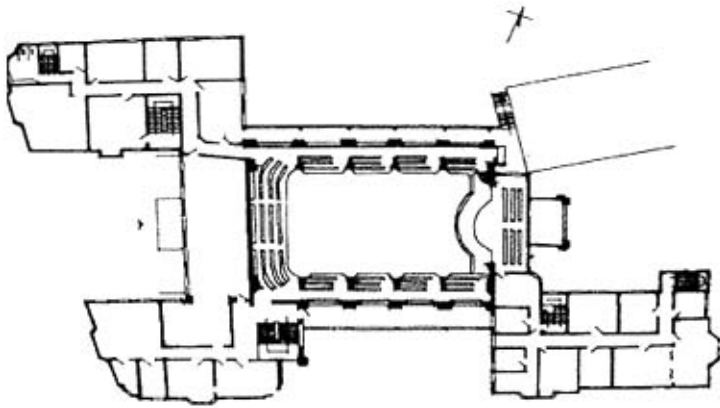
图 4.9 慕尔堂平面图
