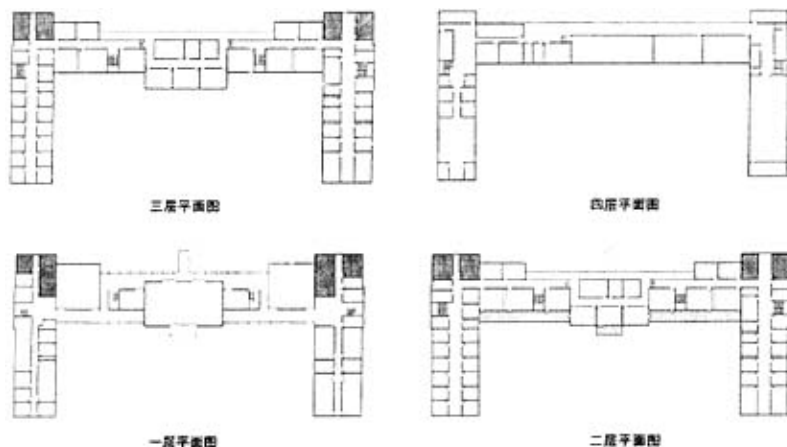
图 4.14 海涵堂平面图
