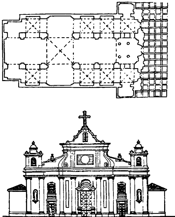
图 3.15 董家渡天主堂平面和立面
