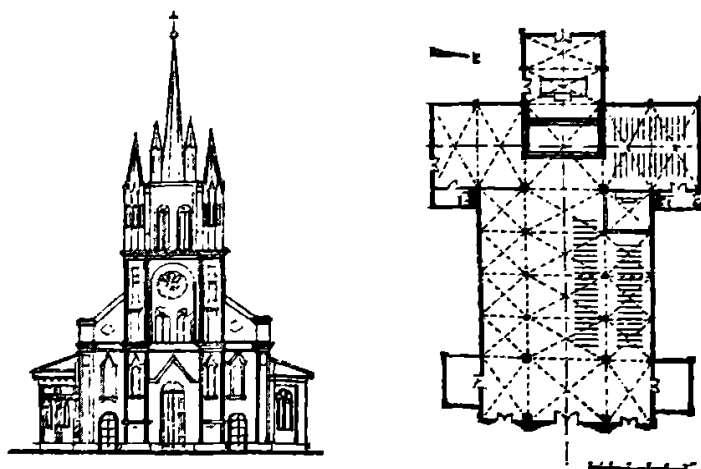
图 3.16 洋泾浜天主堂平面和立面
